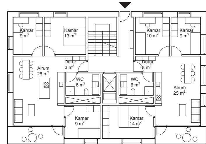
2. OG 3. HÆDD (1:200)
