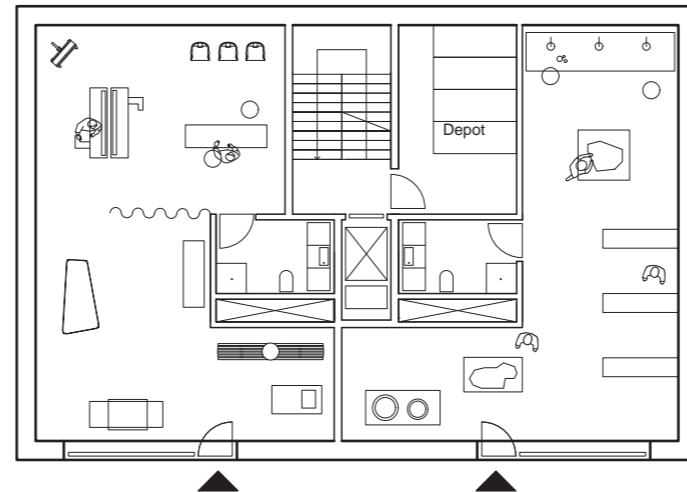
1. HÆDD (1:200)
