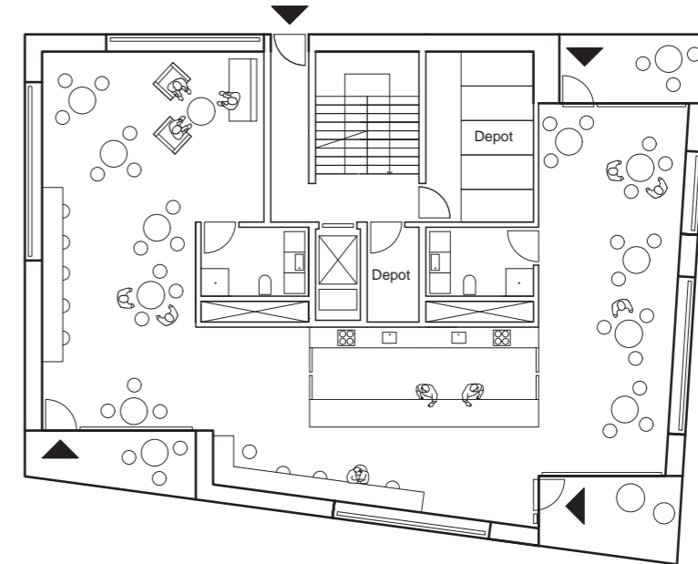
1. HÆDD (1:200)
