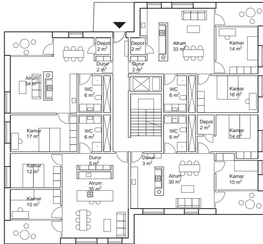
1.-3. HÆDD (1:200)
